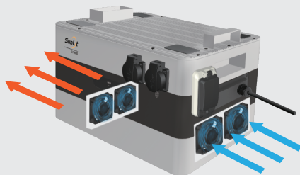
Abbildung 4-4 Luftgekühlte Wärmeableitung
